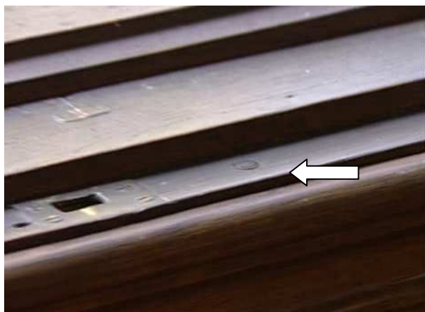
Magnetický kontakt v rámu okna
