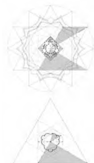
PUBLIKACE OBSAHUJE CELKEM 564 VÝKRESŮ A FOTOGRAFIÍ. NA SNÍMCÍCH JEDNOTLIVÁ MĚŘENÍ KE KOSTELU SV. JANA NEPOMUCKÉHO VE ŽĎÁRU NAD SÁZAVOU
