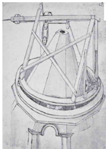
BONACCORSO Ghiberti, SKICA ROTAČNÍHO JEŘÁBU, RUKOPIS ZIBALDONE, FLORENCIE
